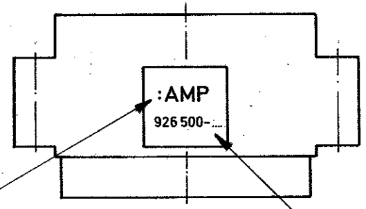
MITTELSCHRIFT 3 DIN 1451
