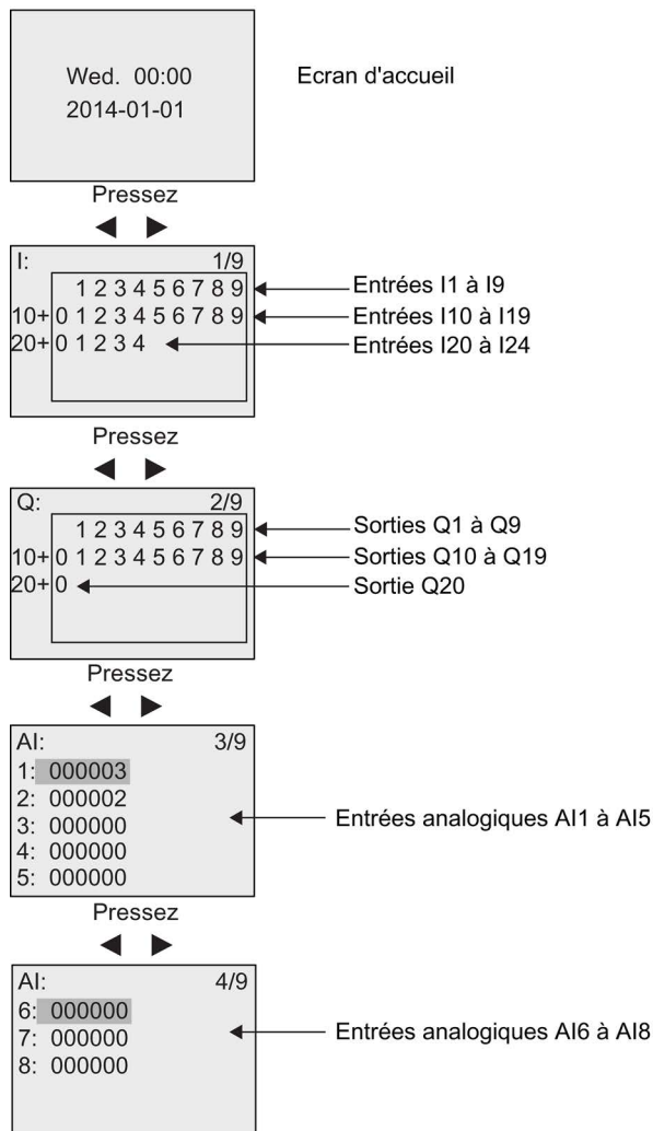
Ecran d'affichage de LOGO! à l'état de fonctionnement RUN
