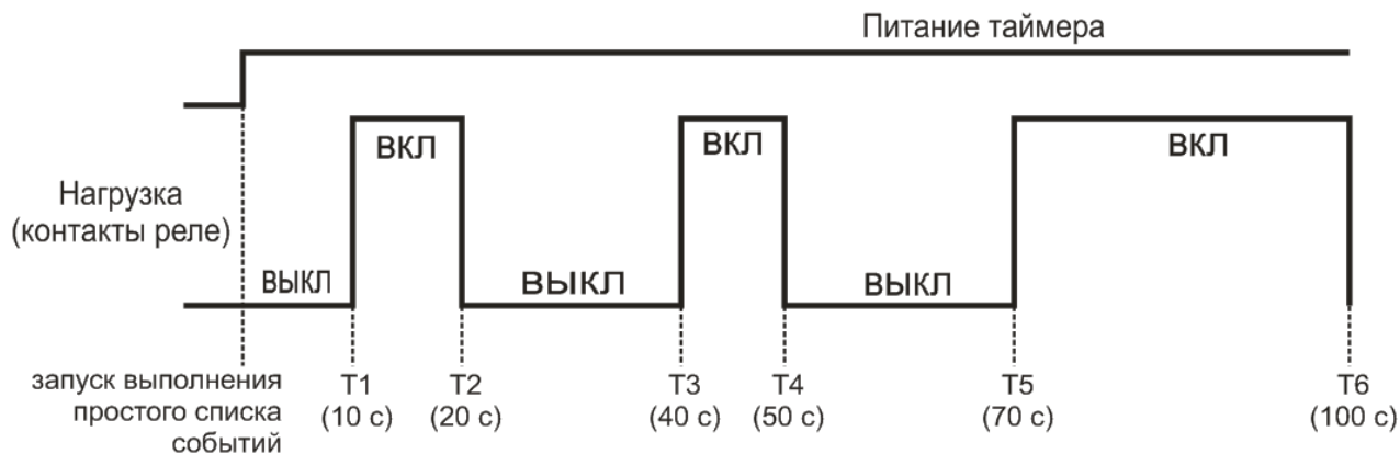
Рисунок 3.6 – Включение нагрузки на примере простого режима работы
