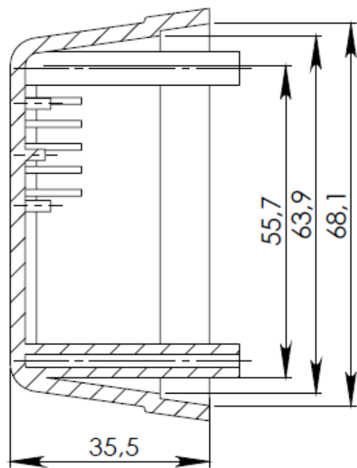
PRZEKRÓJ A-A SKALA 1 : 1
