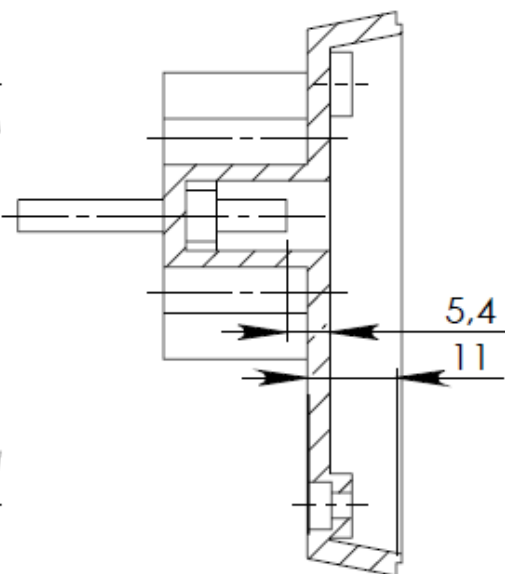
PRZEKRÓJ B-B SKALA 1 : 1
