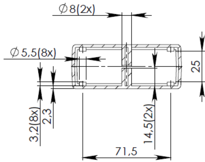
PRZEKRÓJ A-A
