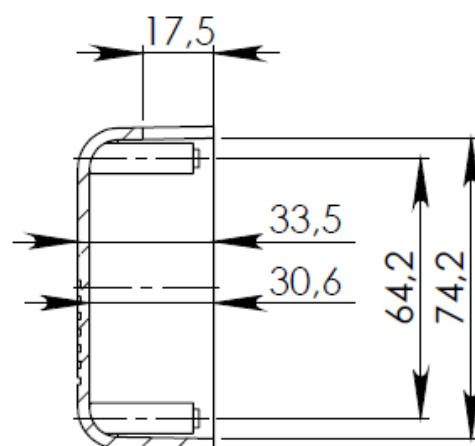
PRZEKRÓJ B-B
