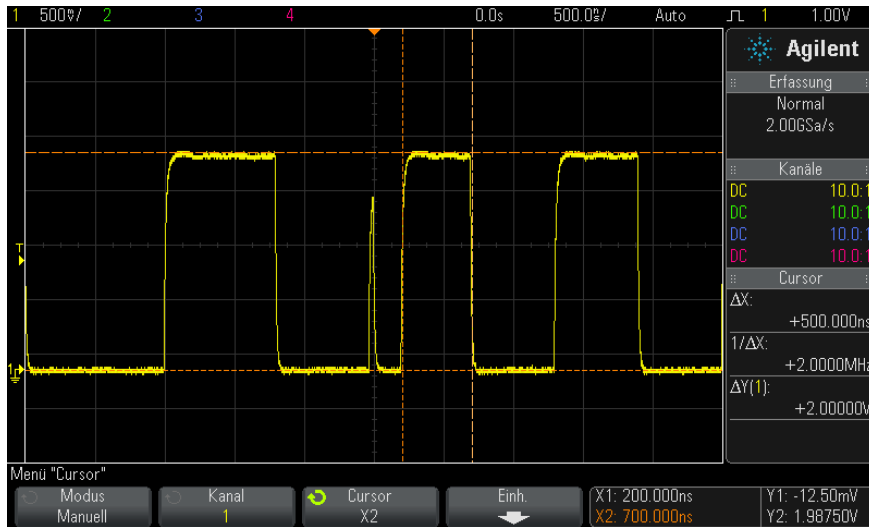
Abbildung 31 Impulsbreitenmessung mithilfe von Cursors
