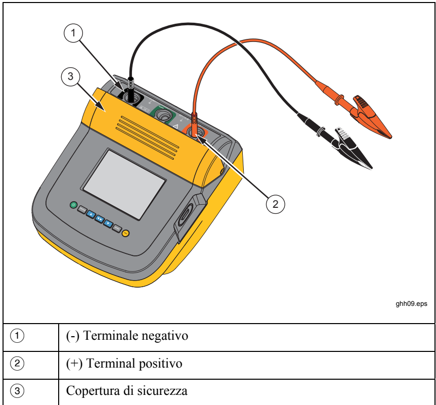
Figura 9. Connessioni dei cavetti di prova
