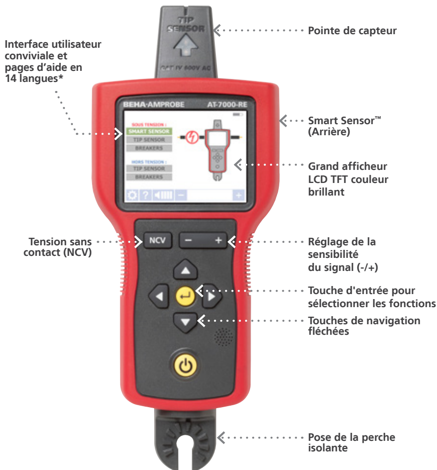
Récepteur AT-7000-RE
