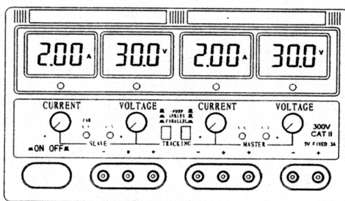
Ilustracja 4-3 (Wyświetlacze LCD)
