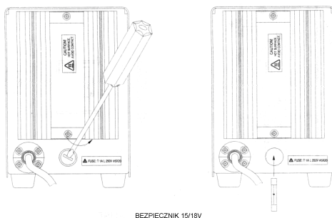
BEZPIECZNIK 15/18V
