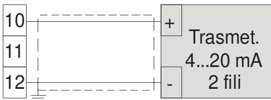
Fig. 8 Collegamento di segnali 0/4-20 mA a trasmettitore passivo con alimentazione ausiliaria
