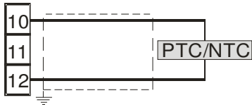
Abb. 6 Anschluss von Thermistoren
