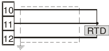
Abb. 5 Anschluss von Widerstandsthermometern
