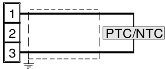
Fig. 6 Connexion de thermisteur
