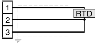
Fig. 5 Connexion de thermorésistance
