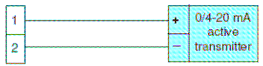
Fig. 6 Cableado 0/4-20 mA para transmisor activo
