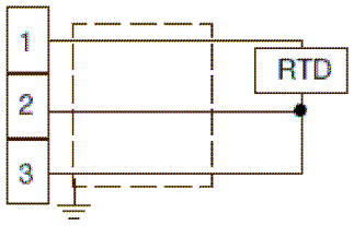
Fig. 5 Cableado RTD (Pt100)
