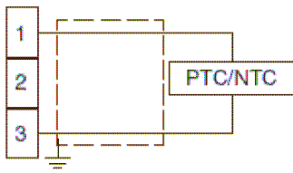
Fig. 6 Cableado PTC / NTC
