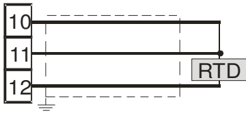
Fig. 5 Cableado RTD (Pt100)
