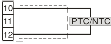
Fig. 6 Cableado PTC / NTC
